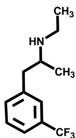
Fenfluramine (8)
